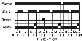
Config. 9 Hafızalı olarak enerji ile birlikte zamanlama +TOFF zamanından sonra START ile reset
