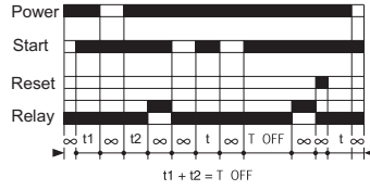
Config. 1 Enerji ile birlikte gecikme verme
